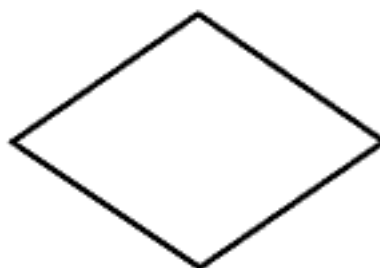
Rhombus
